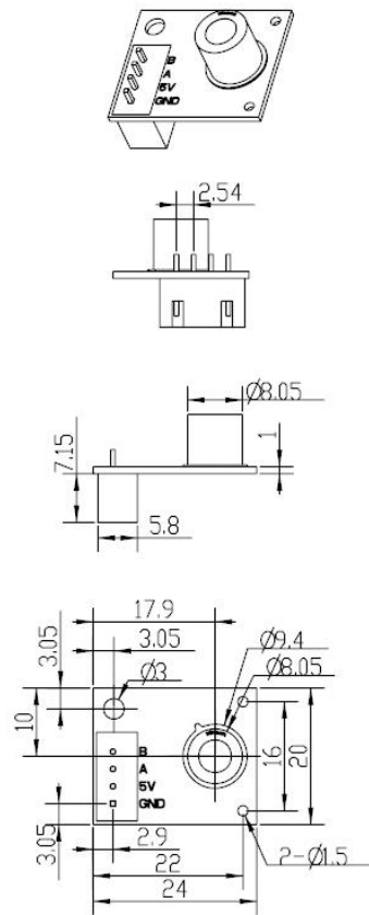
图 1: 模组结构图
